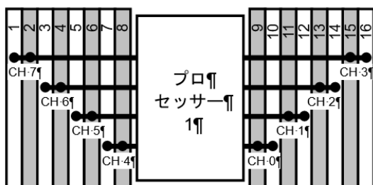
StoreEasy 1870 Storage のプロセッサとメモリスロットのレイアウト
