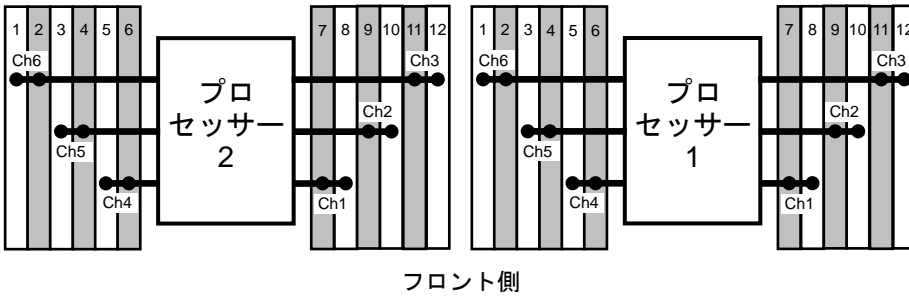
StoreEasy 1660 のプロセッサとメモリ スロットのレイアウト
