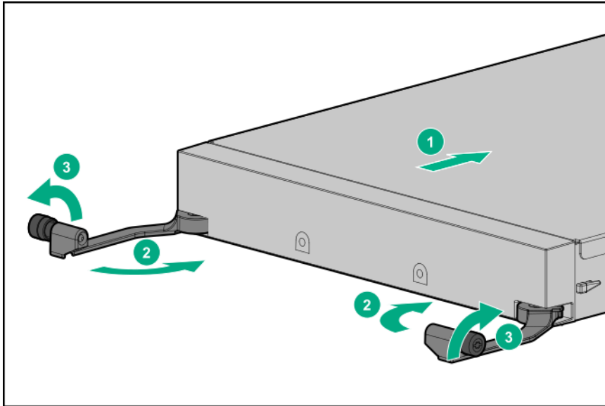
図 2: I/O モジュールの取り付け、ドライブエンクロージャー
