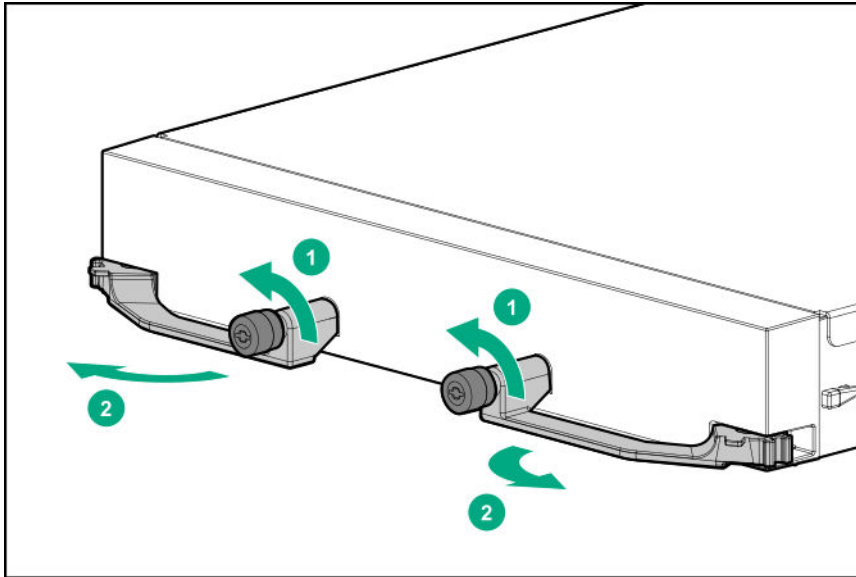
図 1: I/O モジュールの取り外し、ドライブエンクロージャー
