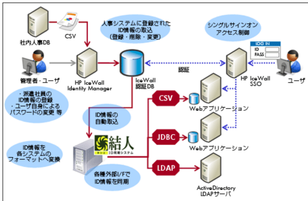
HP IceWall SSOと結人との連携例
