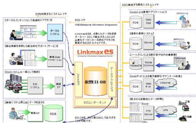
図 1 Linkmax EII Serverが実現するシステムイメージ
