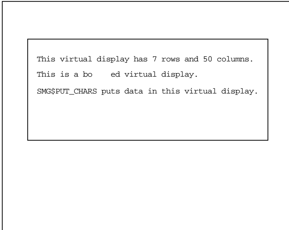
図 8-18 SMG$ERASE_CHARS ルーチン呼び出した後に生成される出力
