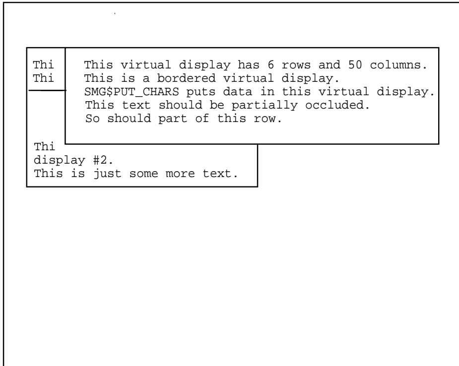
図 8-7 SMG$COPY_VIRTUAL_DISPLAY ルーチン呼び出し後に生成される出力
