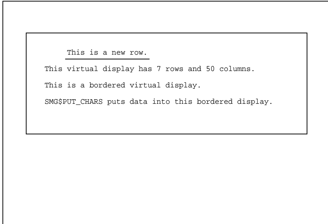
図 8-25 SMG$INSERT_CHARS ルーチンを実行した後に生成される出力
