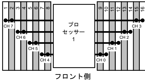
ProLiant ML110 Gen11 サーバーのプロセッサとメモリ スロットのレイアウト
