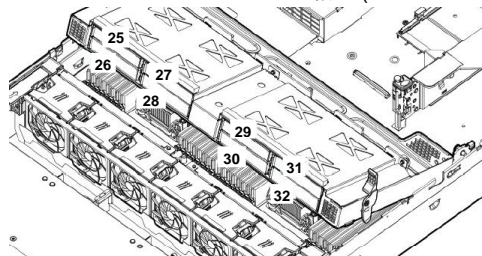
24SFF + ミッドプレーン 8SFF 構成(オプション)
