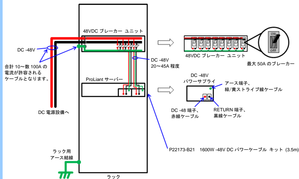
48VDC ブレーカー ユニットを使用した 1600W DC-48V パワーサプライの DC 配線例
