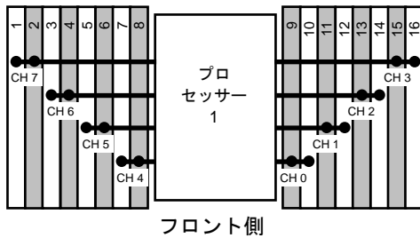
フロント側 ProLiant DL320 Gen11 サーバーのプロセッサとメモリ スロットのレイアウト
