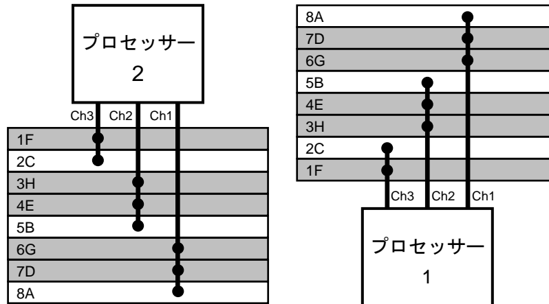
HP ProLiant SL170s G6 サーバートレイの プロセッサとメモリ スロットのレイアウト
