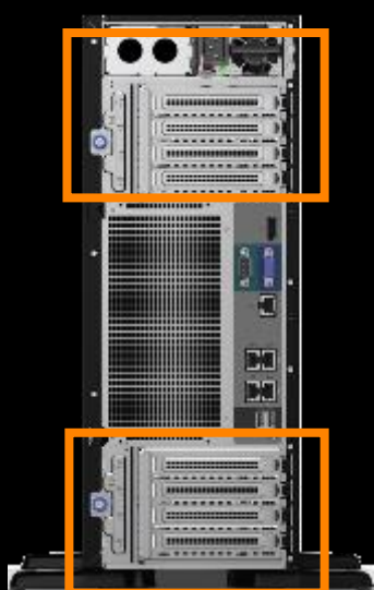
ML350 Gen10 (背面図)
