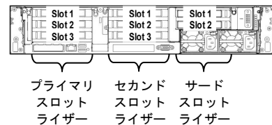
PCI スロット ライザー搭載位置
