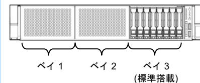
前面ドライブベイ搭載位置
