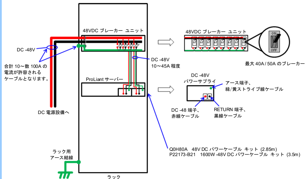
48VDC ブレーカー ユニットを使用した 800W / 1600W DC-48V パワーサプライの DC 配線例
