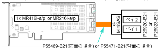
ドライブケージ、ケーブル、コントローラー 接続イメージ図
