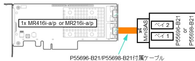
ドライブケース、コントローラー、ケーブル 接続イメージ図
