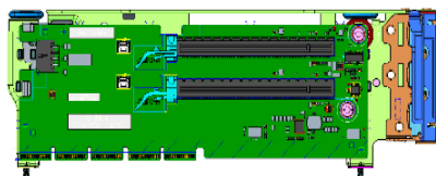
Slot2-3 セカンド スロット ライザー (2x16)
