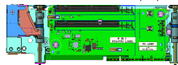
サード スロット ライザー (2x8)
