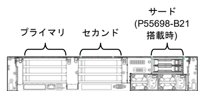
背面ドライブベイ搭載位置
