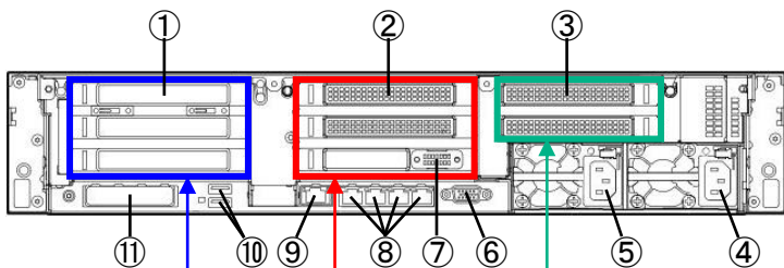
プライマリ PCI スロット ライザー (標準搭載) セカンド PCI スロット ライザー (オプション) サード PCI スロット ライザー (オプション)
