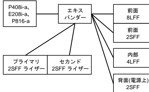
8LFF モデル 12LFF+8SFF 構成
