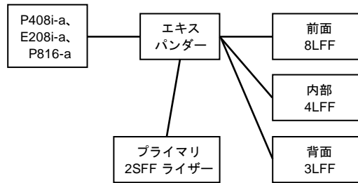
8LFF モデル 15LFF+2SFF 構成
