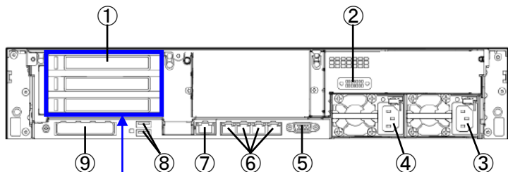
プライマリ PCI スロット ライザー (標準搭載)
