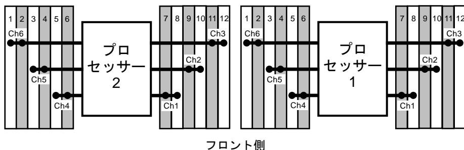
ProLiant DL380 Gen10 サーバーのプロセッサとメモリ スロットのレイアウト
