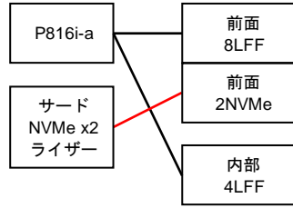
8LFF モデル 12LFF+2NVMe 構成
