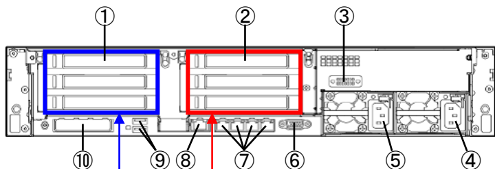
プライマリ PCI スロット ライザー (標準搭載) セカンド PCI スロット ライザー (オプション)
