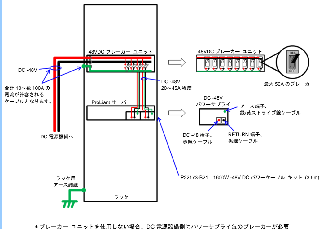
48VDC ブレーカー ユニットを使用した 1600W DC-48V パワーサプライの DC 配線例
