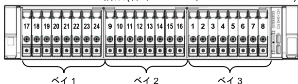
24SFF 構成(標準 8SFF+オプション 8SFFx2)
