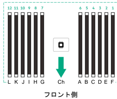
ProLiant DL345 Gen11 サーバーのプロセッサとメモリ スロットのレイアウト
