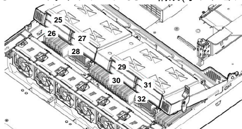
24SFF + ミッドプレーン 8SFF 構成(オプション)
