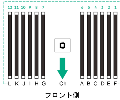
ProLiant DL325 Gen11 サーバーのプロセッサとメモリ スロットのレイアウト
