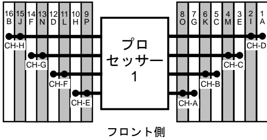
フロント側 ProLiant DL325 Gen10 Plus v2 サーバーのプロセッサとメモリ スロットのレイアウト
