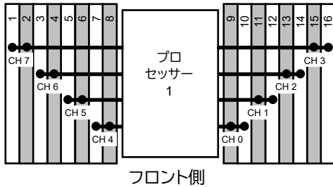
フロント側 ProLiant DL320 Gen11 サーバーのプロセッサとメモリ スロットのレイアウト
