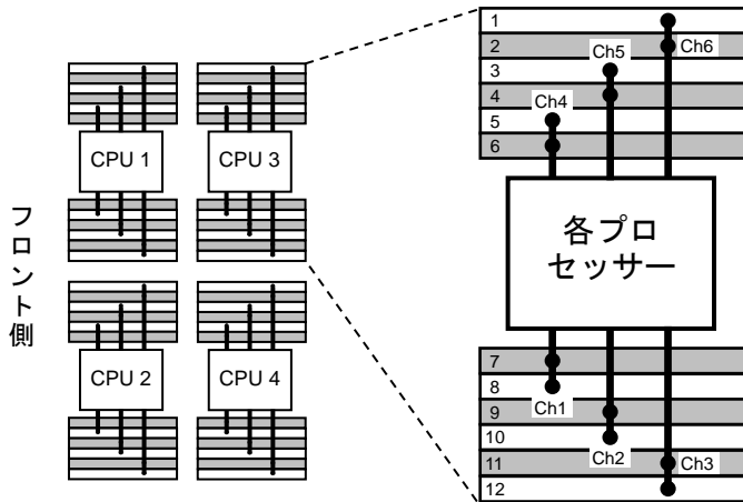
Synergy 660 Gen10 コンピュート モジュールの プロセッサーとメモリ スロットのレイアウト
