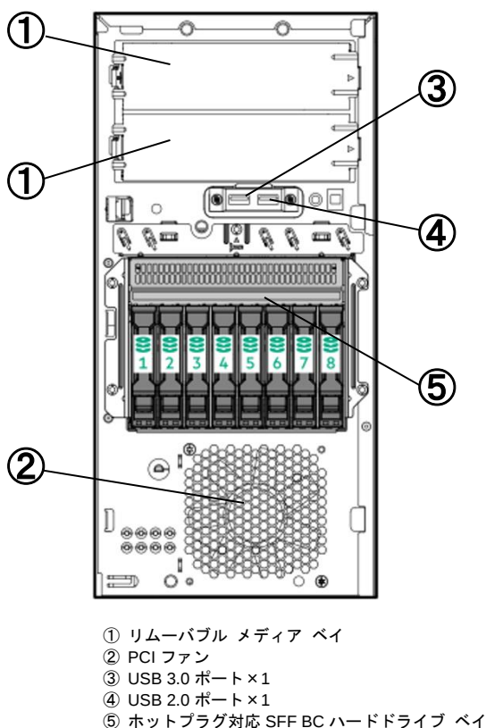
ホットプラグ SFF モデル前面図
