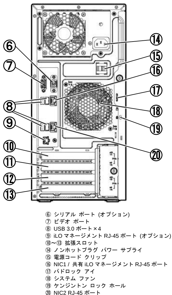
全モデル共通 背面図
