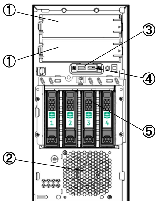
ホットプラグ LFF モデル前面図
