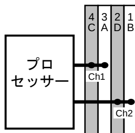
ProLiant ML30 Gen10 Plus サーバーの プロセッサとメモリ スロットのレイアウト
