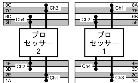
ProLiant ML150 Gen9 サーバーのプロセッサとメモリ スロットのレイアウト
