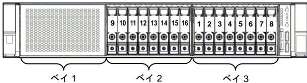
16SFF 構成(標準前面)
