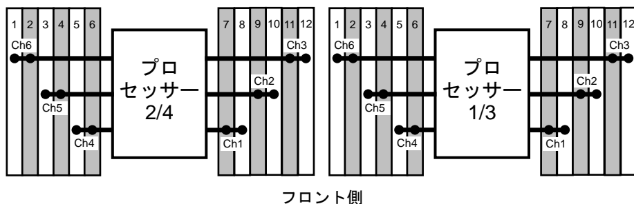
ProLiant DL560 Gen10 サーバーのプロセッサとメモリ スロットのレイアウト
