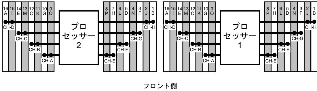
ProLiant DL385 Gen10 サーバーのプロセッサとメモリ スロットのレイアウト
