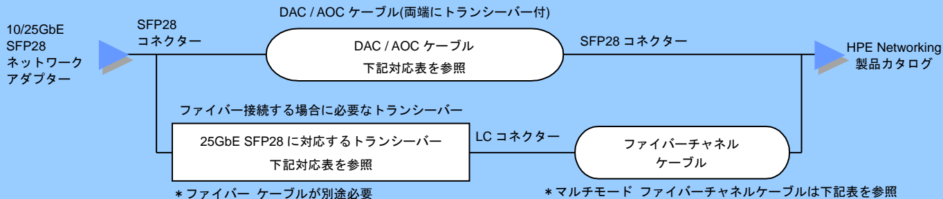
マルチモード ファイバーチャネル ケーブル (LC-LC)
