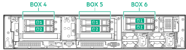
オプション 2SFFx3 (背面)
