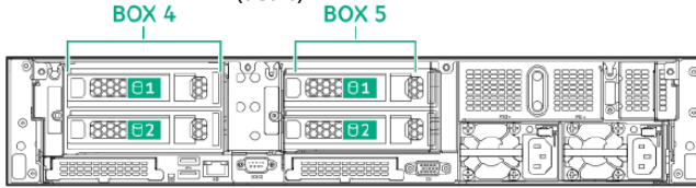
標準 12LFF
