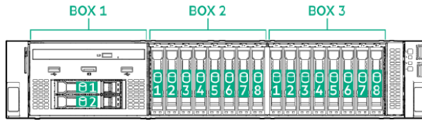
前面 SFF ドライブケース搭載位置
