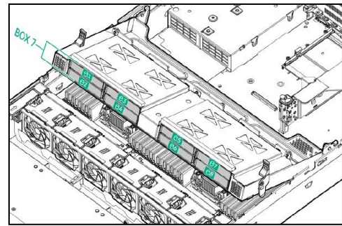
オプション 8SFF (ミッドトレイ)
