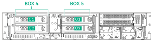
背面 LFF ドライブケース搭載位置
