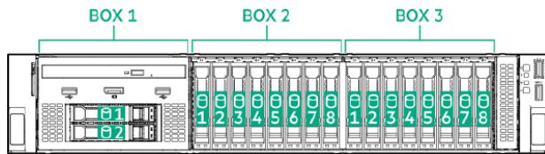
前面 SFF ドライブケース搭載位置
