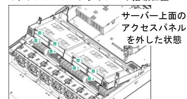
ミッドプレーン ドライブベイ搭載位置
