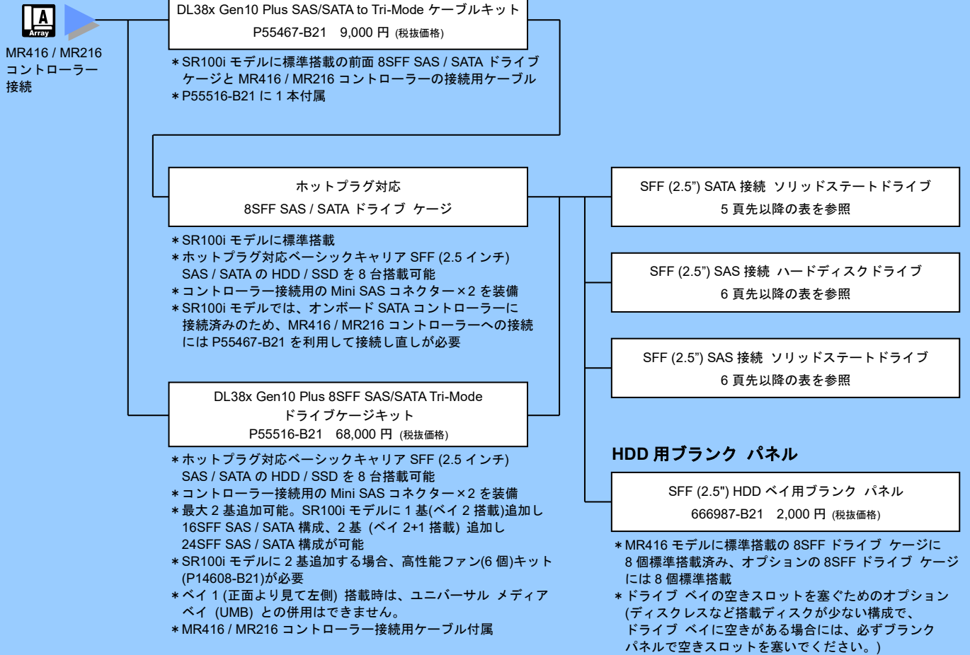
ドライブケース、コントローラー、 ケーブル 接続イメージ図
