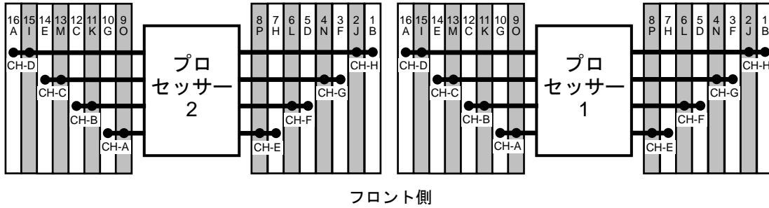
ProLiant DL365 Gen10 Plus サーバーのプロセッサとメモリ スロットのレイアウト
