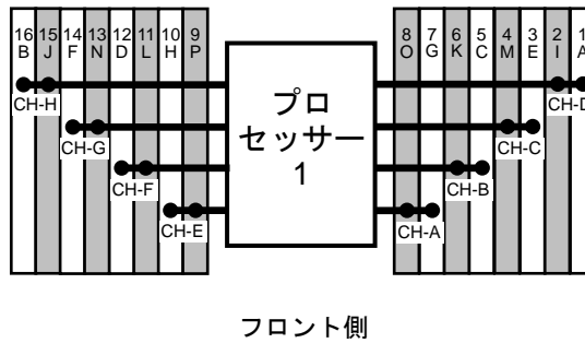
ProLiant DL325 Gen10 サーバーのプロセッサとメモリ スロットのレイアウト
