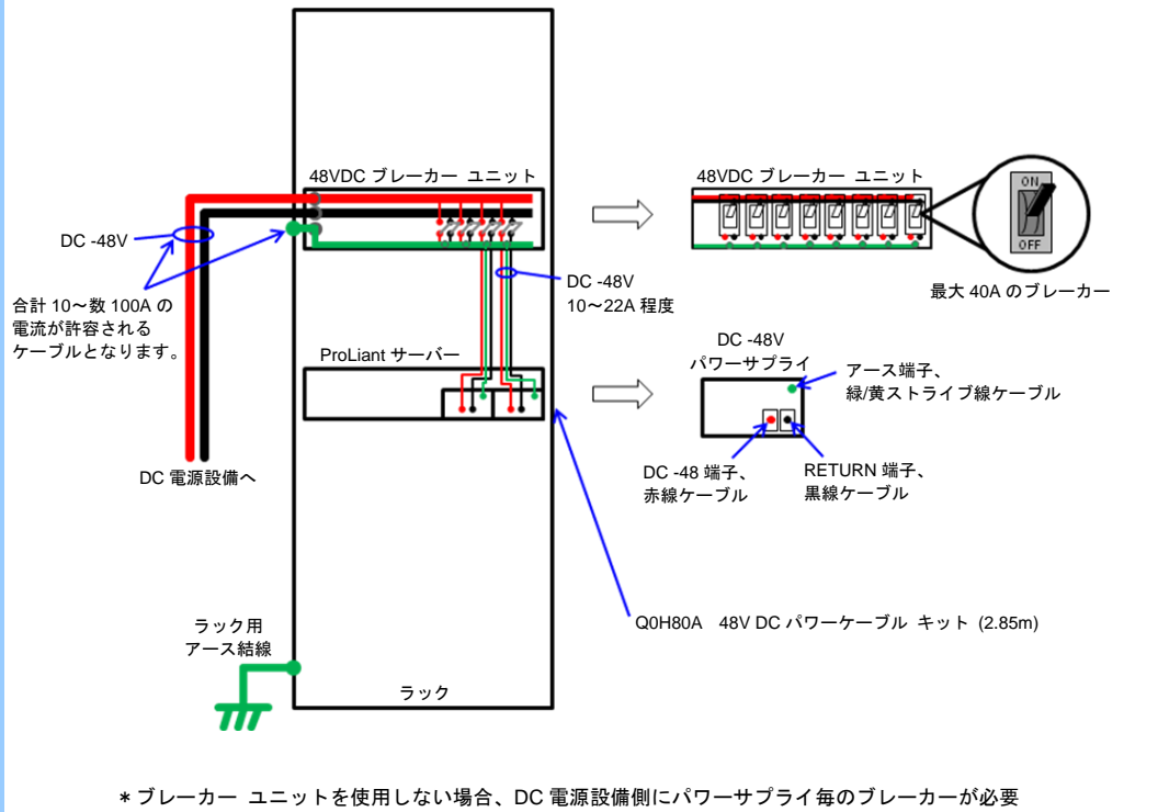
48VDC ブレーカー ユニットを使用した 800W DC-48V パワーサプライの DC 配線例
