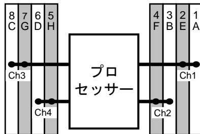
ProLiant DL120 Gen9 サーバーのプロセッサとメモリ スロットのレイアウト
