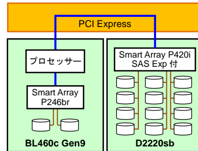
D2220sb ストレージブレードと BL460c Gen9 サーバーブレードの PCI Express 接続
