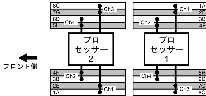
HPE ProLiant BL460c Gen9 サーバーブレードのプロセッサとメモリ スロットのレイアウト
