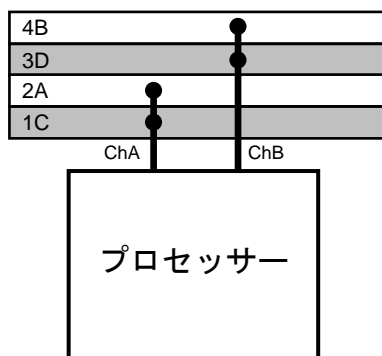
HP ProLiant ML110 G7 サーバーの プロセッサーとメモリ スロットのレイアウト
