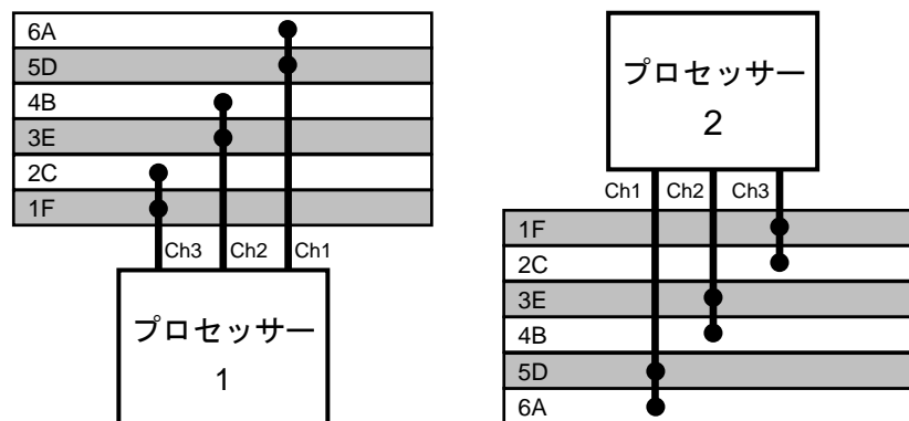
HP ProLiant SL390s G7 4U サーバートレイの プロセッサとメモリ スロットのレイアウト
