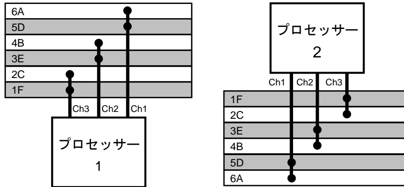
HP ProLiant SL390s G7 2U サーバートレイの プロセッサとメモリ スロットのレイアウト
